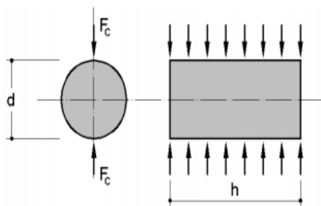
Figura 2.3 – Ensaio de tração por compressão diametral
