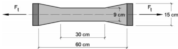
Figura 2.2 – Ensaio de tração direta
